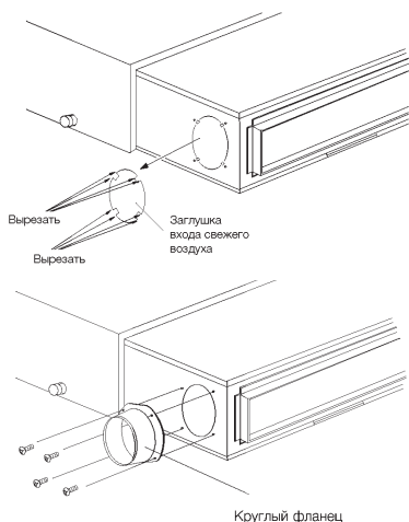
Круглый фланец
